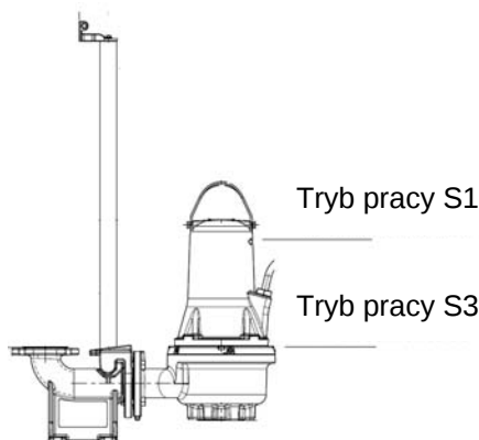
Rys. 2 Poziomy wyłączania
