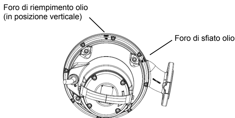
Fig. 11 Fori di riempimento dell'olio
