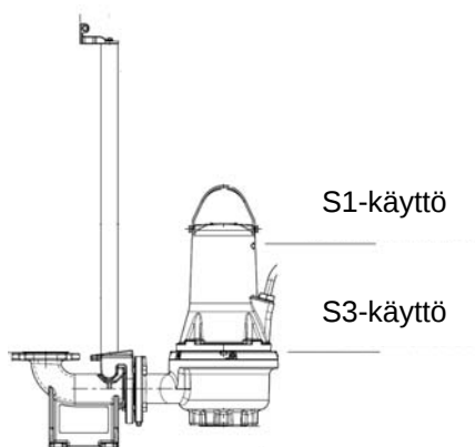
Kuva 2 Pysäytystasot
