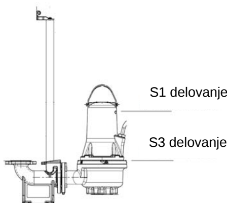
Slika 2 Izklopni nivoji
