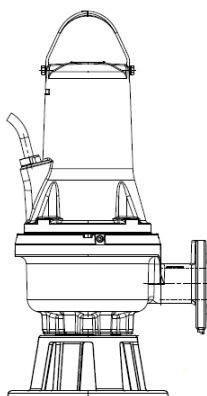
Fig. 7 Fristående dränkt installation på ringstativ
