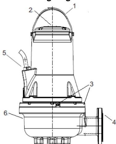
Fig. 1 FK -pumpe
