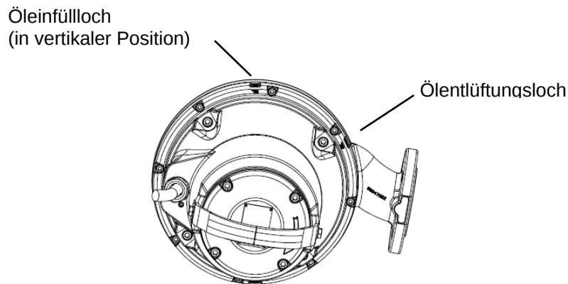
Abb. 11 Öleinfüllöffnungen
