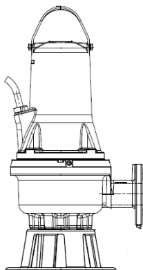
Fig. 7 Installation immergée autonome sur socle circulaire
