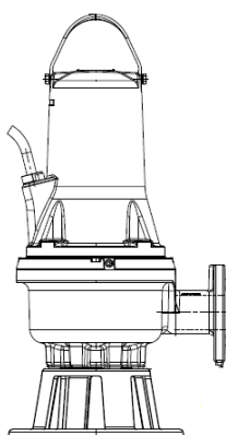
Joonis 7 Vabalt seisev sukelpaigaldus kinnitusega ringalusele
