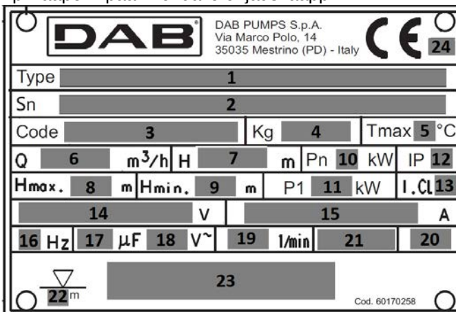
Kuva 3 Tyypikilpi
