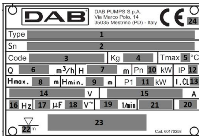
Slika 3 Natpisna pločica
