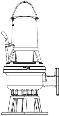
Şekil 7 Halka stand üzerine desteksiz dalgıç kurulumu
