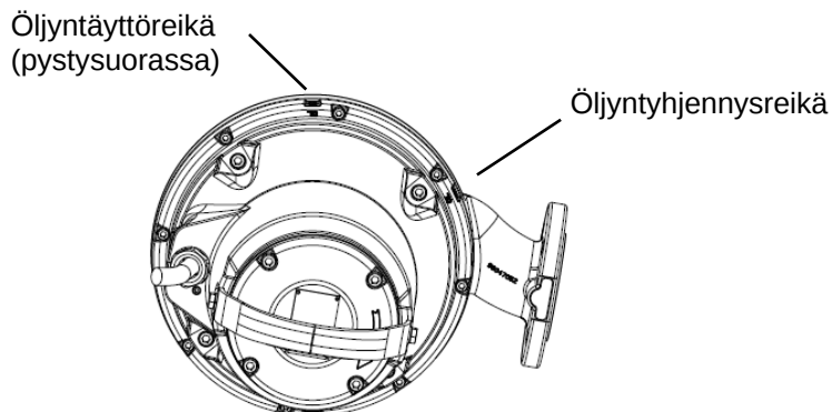
Kuva 11 Öljyn täyttöaukot
