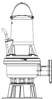
Fig. 7 Instalação portátil submersa
