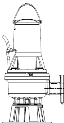
Slika 7 Prostostoječa potopna montaža na obročastem stojalu
