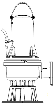
Rys. 7 Wersja montażowa wolnostojąca mokra z podstawą pierścieniową
