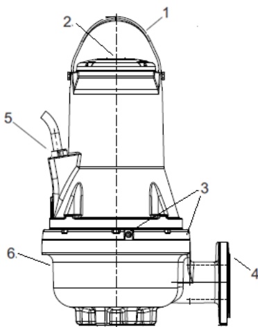
Fig. 1 Bomba FK
