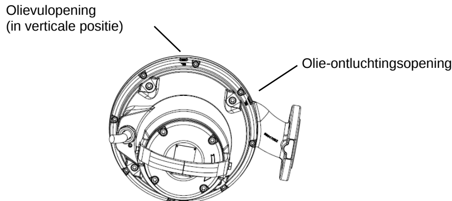
Afb. 11 Olievulopeningen
