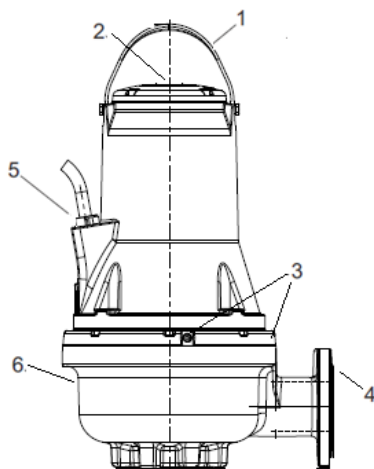
Fig. 1 Pompe FK
