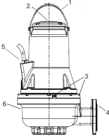
Şekil 1 FK pompası
